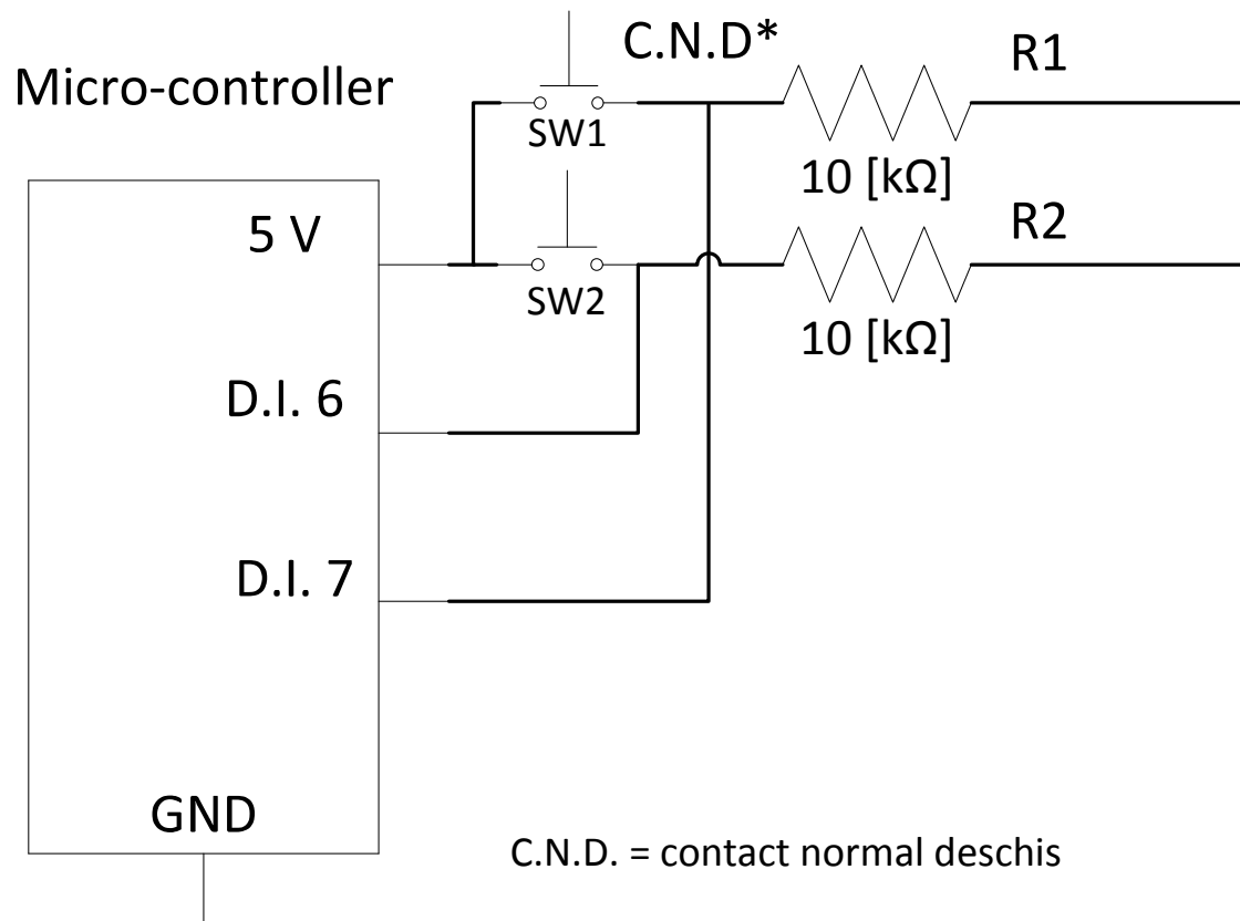
Schemă de principiu – Laborator nr. 2 - „Interacțiunea cu intrările digitale în timp real” (eng. „Digital input real – time interaction”)
