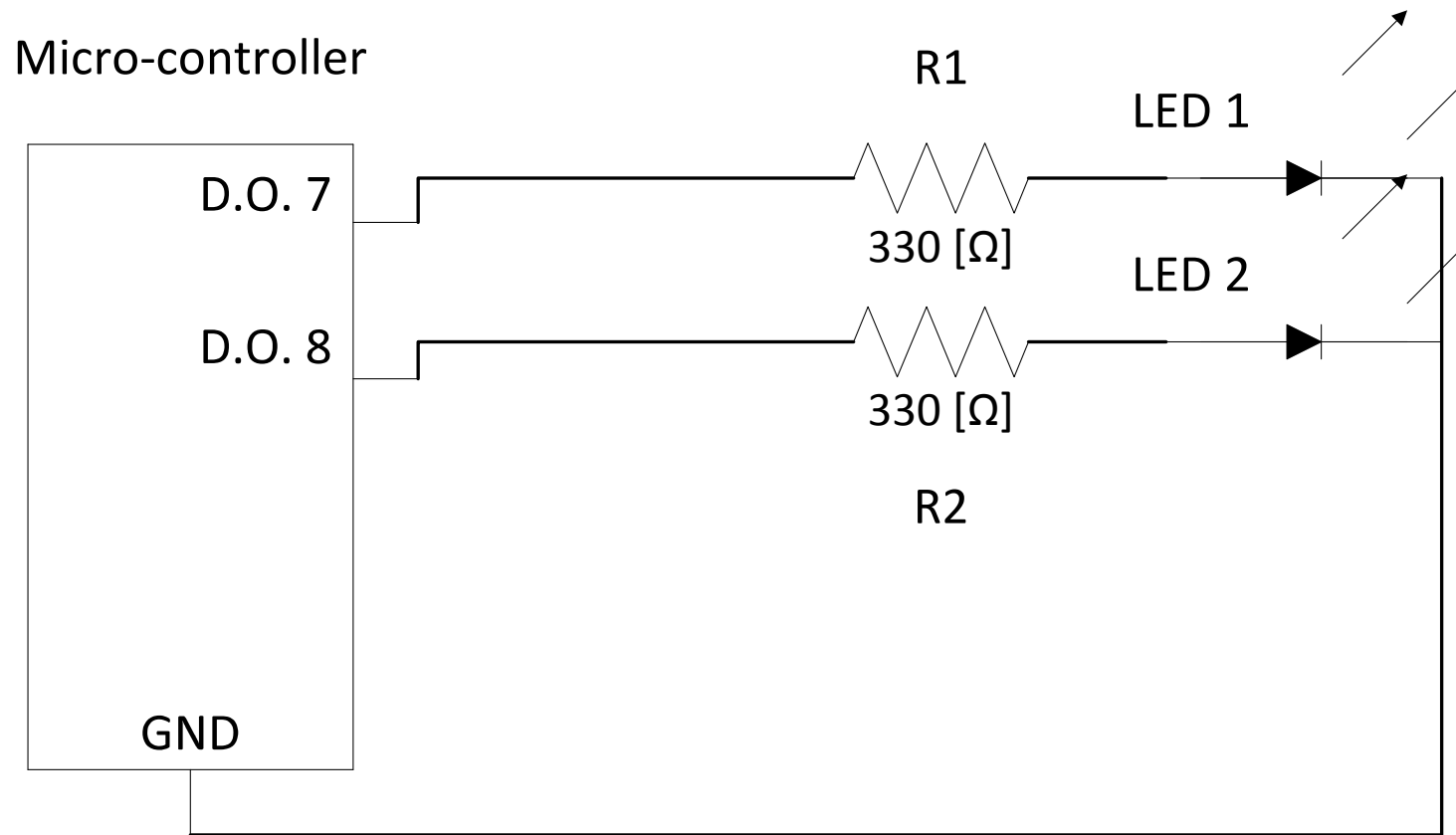
Schemă de principiu – Laborator nr. 1 - „Interacțiunea cu ieșirile digitale în timp real” (eng. „Digital output real – time interaction”)
